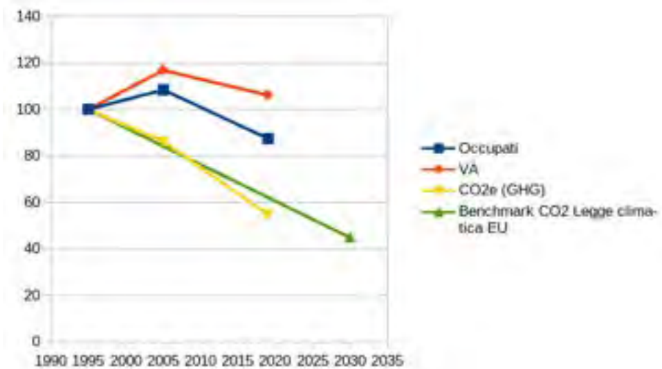
Figura 13: comparazione tra le variazioni 1995-2019 di Occupati, PIL (Val agg) e gas climalteranti nel settore metallurgico (codici C24 e C25 ATECO), (fonte: elaborazione EStà su dati ISTAT)
