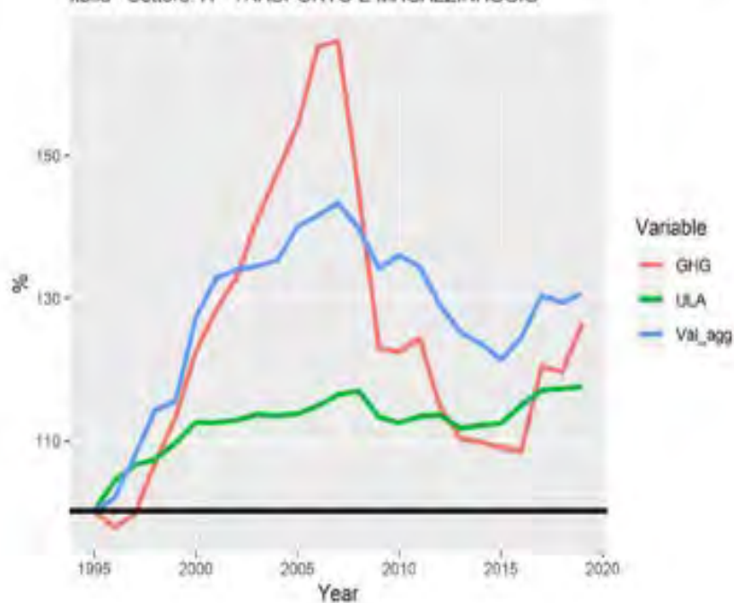
Variazione % dal 1995 al 2020 di GHG, ULA e Valore aggiunto Italia - Settore H - TRASPORTO E MAGAZZINAGGIO
