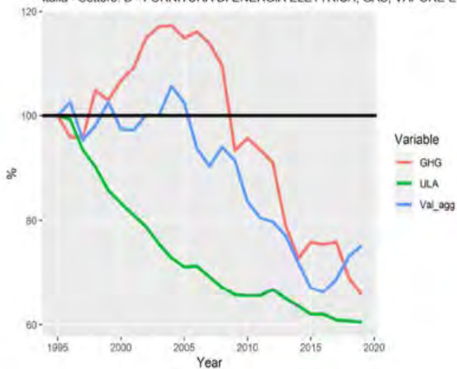
Variazione % dal 1995 al 2020 di GHG, ULA e Valore aggiunto Italia - Settore: D - FORNITURA DI ENERGIA ELETTRICA, GAS, VAPORE E A
