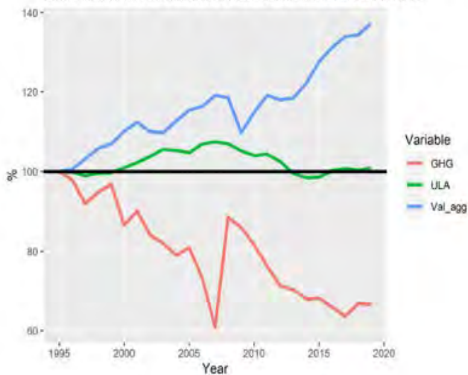
Variazione % dal 1995 al 2020 di GHG, ULA e Valore aggiunto Italia - Settore: G - COMMERCIO ALL'INGROSSO E AL DETTAGLIO
