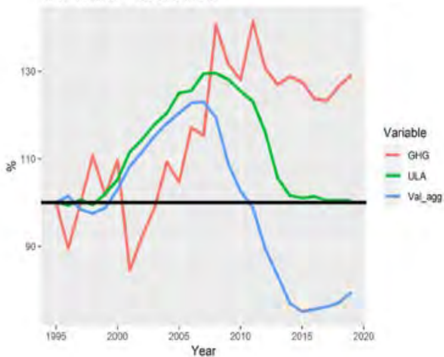
Variazione % dal 1995 al 2020 di GHG, ULA e Valore aggiunto Italia - Settore: F - COSTRUZIONI
