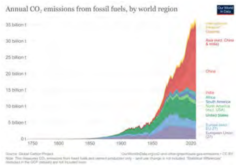
Figura 6: la variazione nel tempo delle aree e dei paesi nel mondo dove si emette più CO 2 (fonte: Our World in data).
