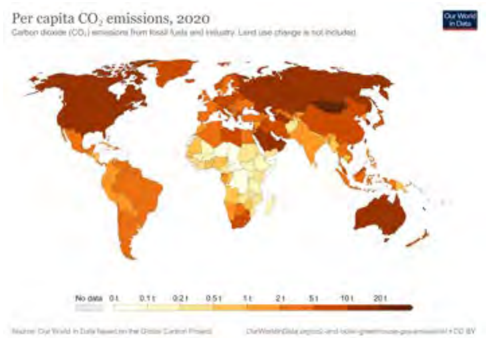
Figura 7: le emissioni mondiali pro capite di CO 2 nel 2020 (fonte: Our World in data). NB Comprende le emissioni di anidride carbonica (CO 2 ) provenienti dalle fonti fossili e dall'industria. Non include gli effetti di cambi d'uso del suolo.
