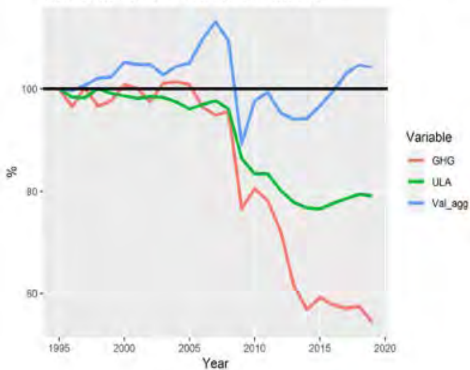
Variazione % dal 1995 al 2020 di GHG, ULA e Valore aggiunto Italia - Settore: C - ATTIVITÀ MANIFATTURIERE
