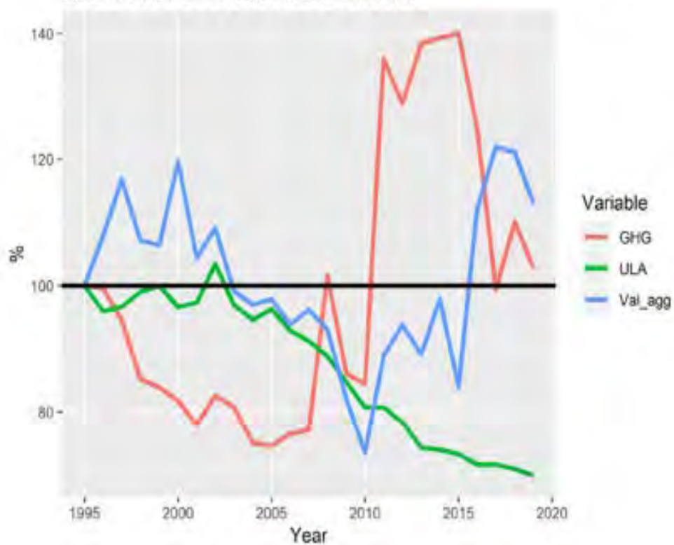
Variazione % dal 1995 al 2020 di GHG, ULA e Valore aggiunto Italia - Settore: B - ATTIVITÀ ESTRATTIVA
